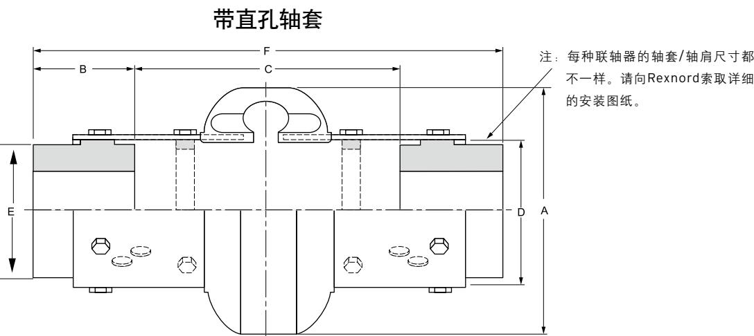
直孔轴套联轴器技术参数
