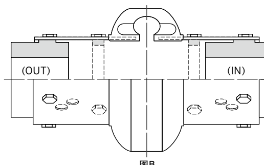
图B 一个轴套向内装 一个轴套向外装
