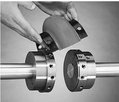
把一个轴套安装在轴上，让另一个轴套处于松动状态以调整间距
