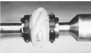
严格的静力试验（5倍额定值）证明了弹性体挠性能力，牢固的结构和金属片与弹性体的结合力。
