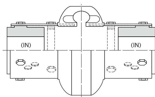
图C 两个轴套都向内装
