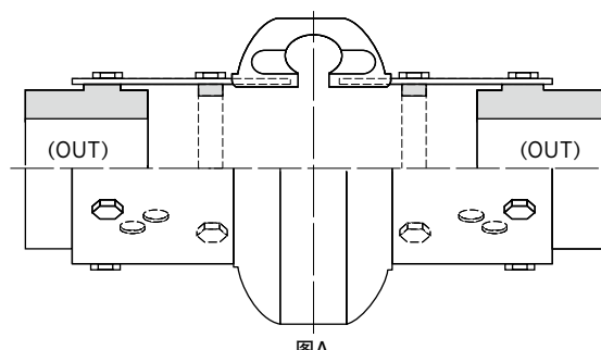
图A 两个轴套都向外装
