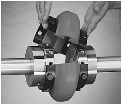
将半个Rexnord® Omega®弹性体安装在轴套上并拧紧自锁螺栓。通过Omega弹性体确定另外一个轴套的间距，再固定那个轴套。
