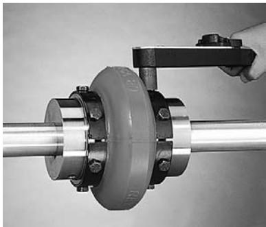
安装另外一半Omega弹性体。拧紧所有螺栓至推荐扭矩就可以了。进一步的细节请参阅安装手册
